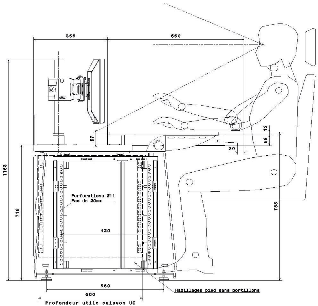
Plan de profil de la console AX®
